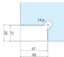
ガラス加工図
