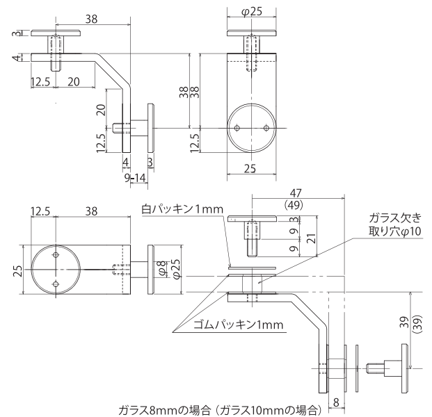
TTS-5058L (ガラス厚8~10mm用) ※専用工具(別売)が必要です。
